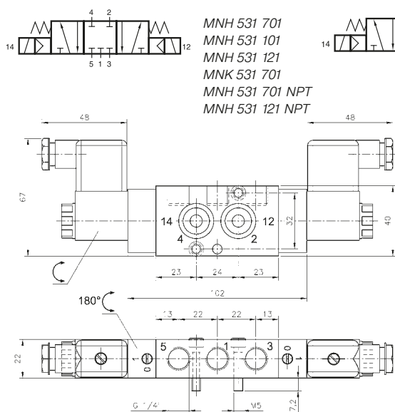
MNH 53_ 701/MNH 531 701 NPT
