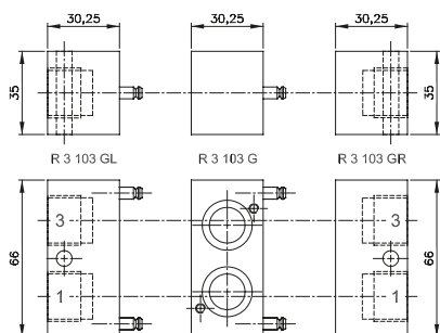
Moduláris alaplapp elemei R 3__ 103 G
