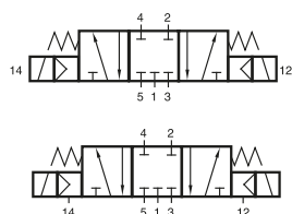
MH 531 501 MH 531 701 MH 531 801
