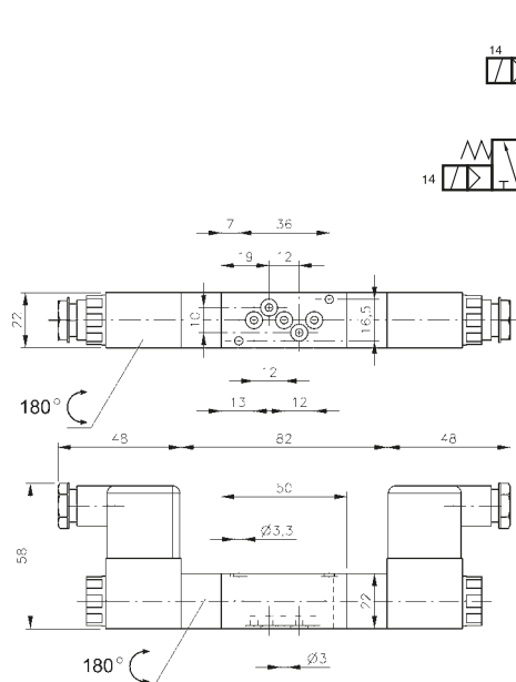
MH 520 304 TT/MH 53_ 304 TT
