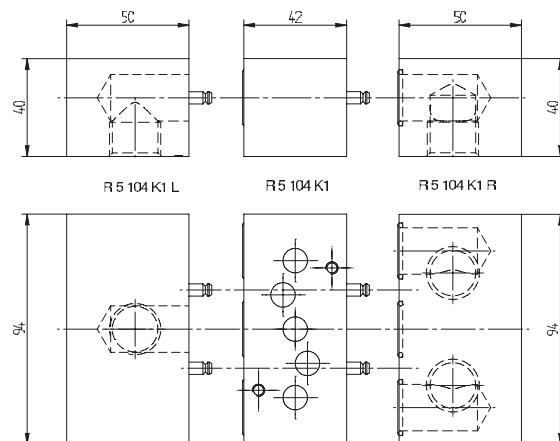
Moduláris alaplap elemei R 5 104 K1
