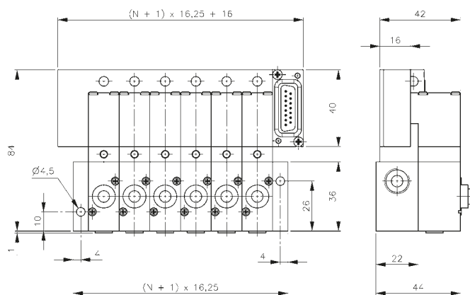
T_16 3__403 463 T típusú szelepekkel
