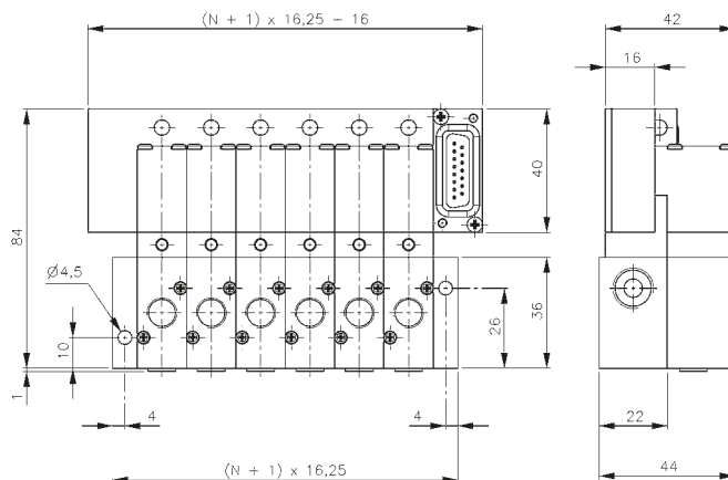
T_16 3__403 403 T típusú szelepekkel
