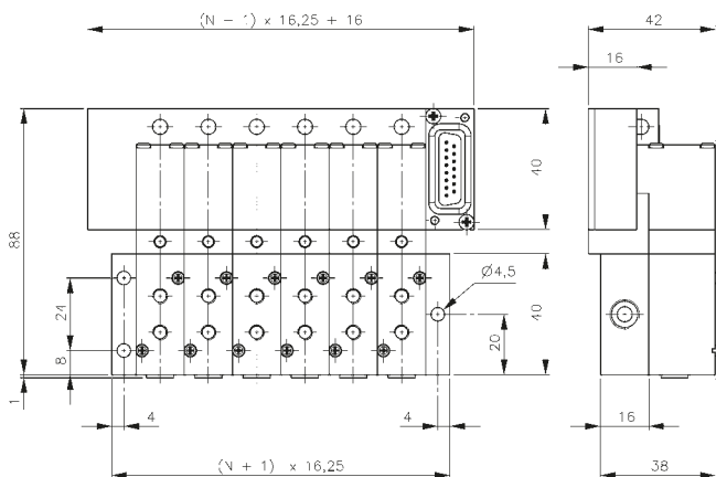
T_16 5__303 303 T típusú szelepekkel felszerelve
