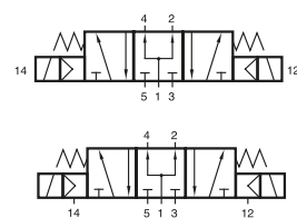
MH 533 501 MH 533 701 MH 533 801
