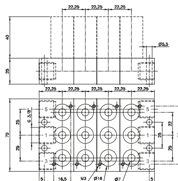
R 5 __ 703 G Furat méret: 15 mm
