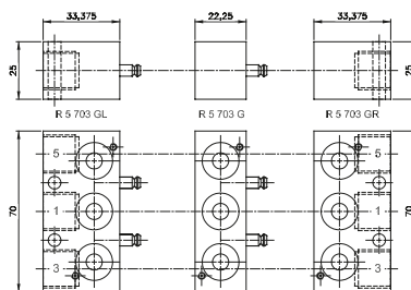
Moduláris alaplap elemei R 5 __ 703 G
