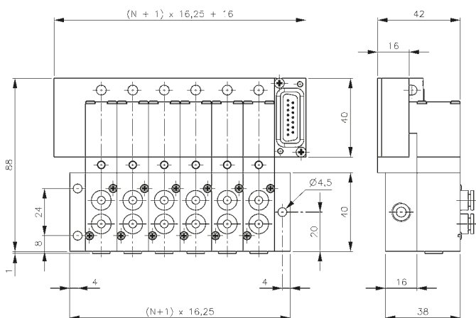
T_16 5__303 343 T típusú szelepekkel
