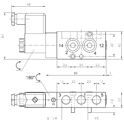
MNH 510 711/MNH 511 711 Csatlakozás 2,4,3,5 felcserélve!
