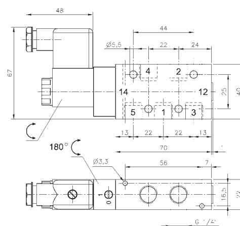
MH 510 701 G TT
