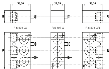
Moduláris alaplapp elemei R 5 __ 503 G
