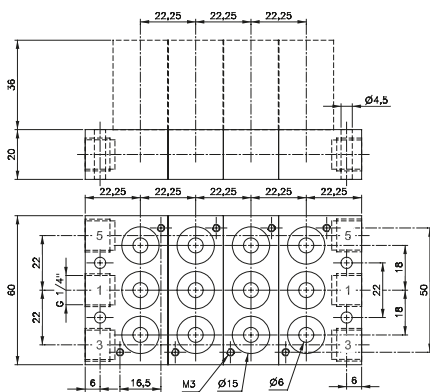
R 5 __ 503 G Furat átmérő: 10 mm
