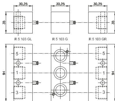
Moduláris alaplapp elemei R 5 __ 103 G
