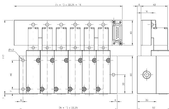
T_22 5_504 504 T típusú szelepekkel felszerelve
