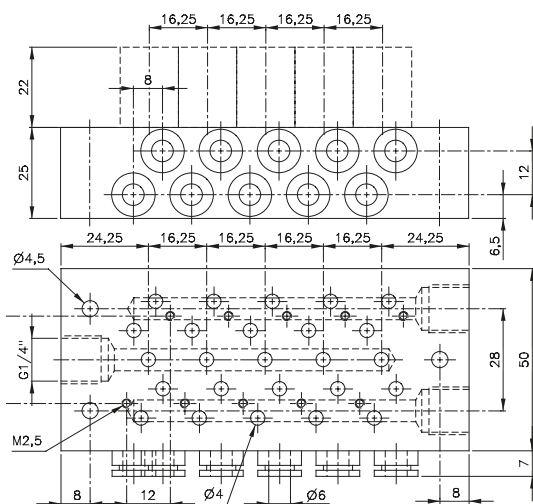
RD 5__ 464 Furat méret: 6 mm
